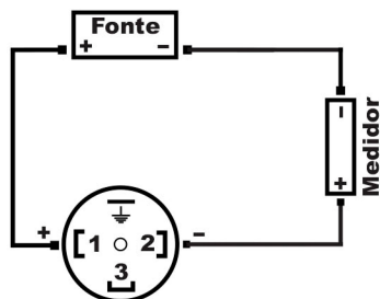
Esquema de Ligação Saída 4/20 mA 2 fios
