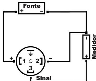
Esquema de Ligação Saída: 0-5, 0-10, 1-5 Vcc - 3 Fios
