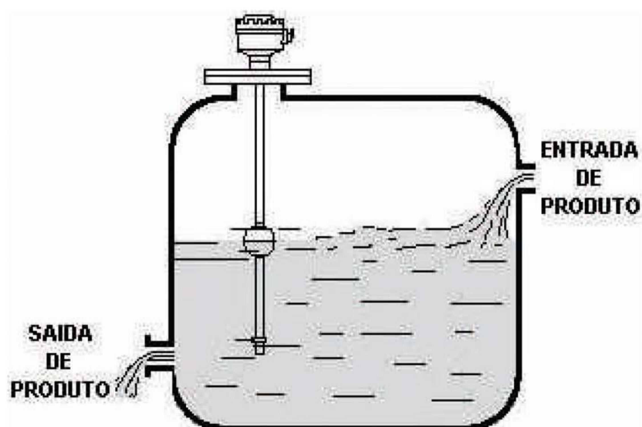
Montagem Topo
